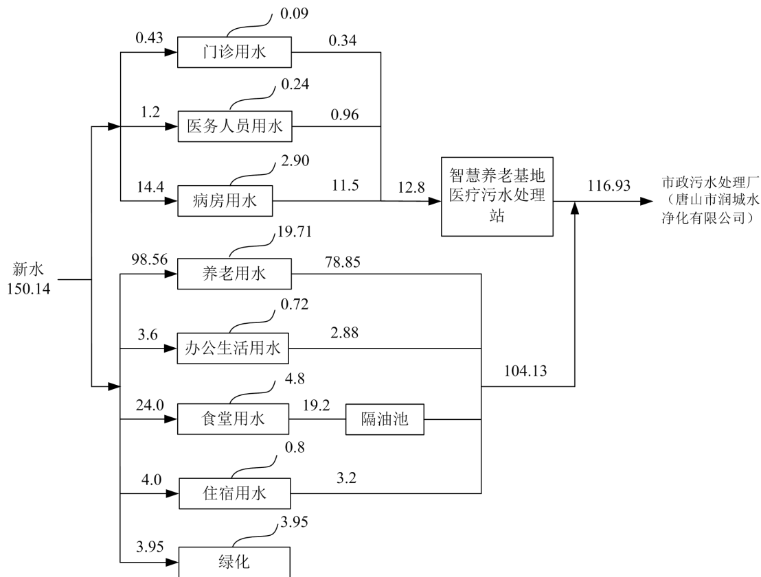
图 2-6 现有智慧养老基地园区水平衡图 单位 \text{m}^3/\text{d}
