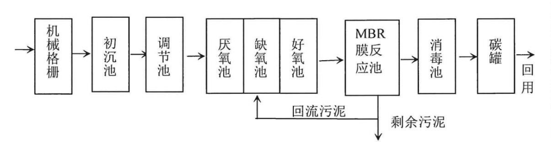
图 2-7 养老服务中心综合污水处理站处理工艺流程图
