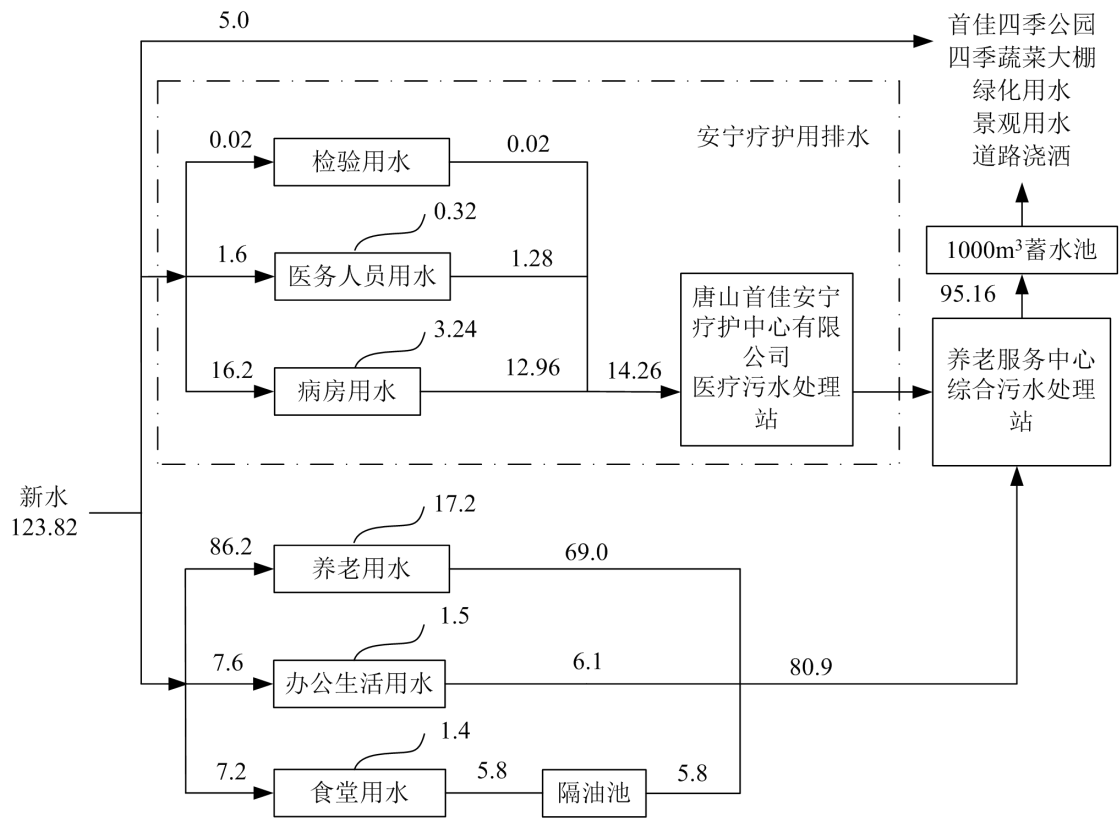
图 2-5 现有养老服务中心水平衡图 单位 \text{m}^3/\text{d}
