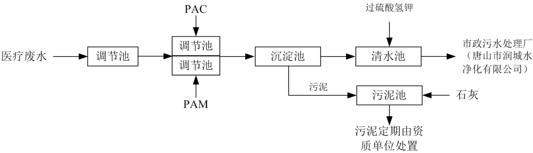
图 2-4 唐山首佳安宁疗护中心有限公司现有医疗污水处理站工艺流程图
