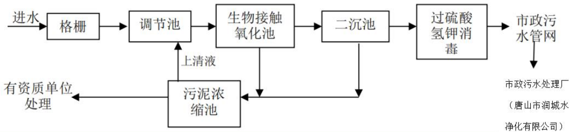
图 2-8 智慧养老基地医疗污水处理站处理工艺流程图
