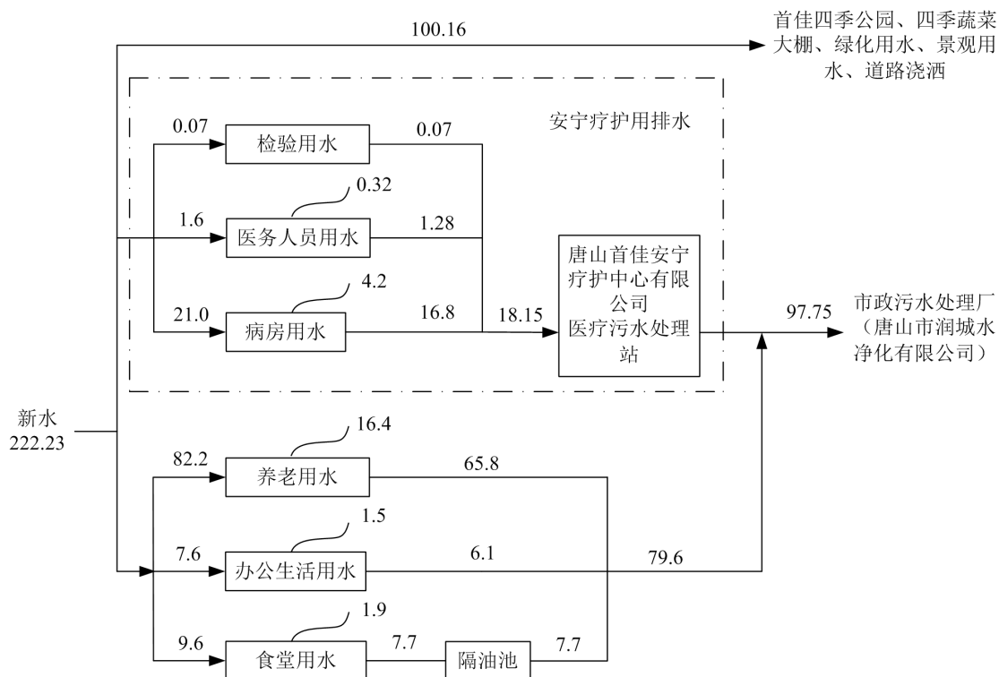
图 2-1 扩建完成后养老服务中心水平衡图（单位：m 3 /d）
