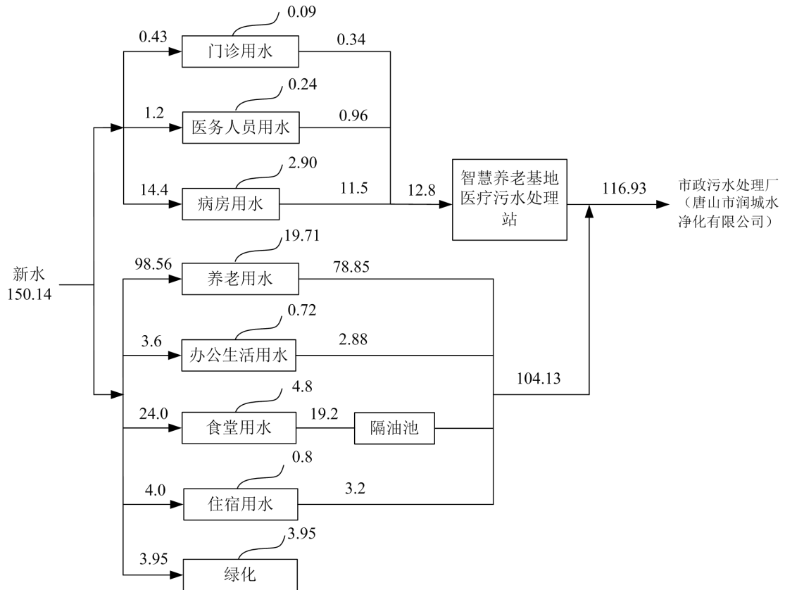
图 2-6 智慧养老基地园区水平衡图 单位 \text{m}^3/\text{d}
