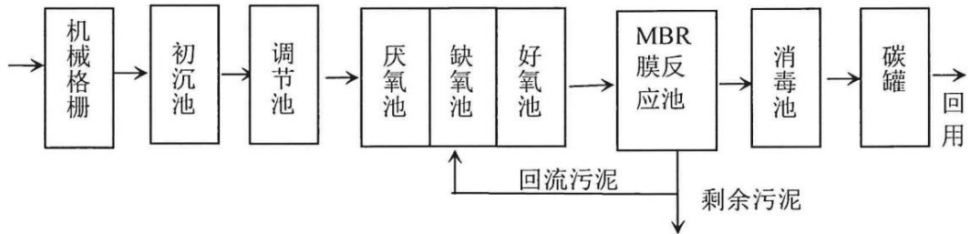
图 2-7 养老服务中心综合污水处理站处理工艺流程图
